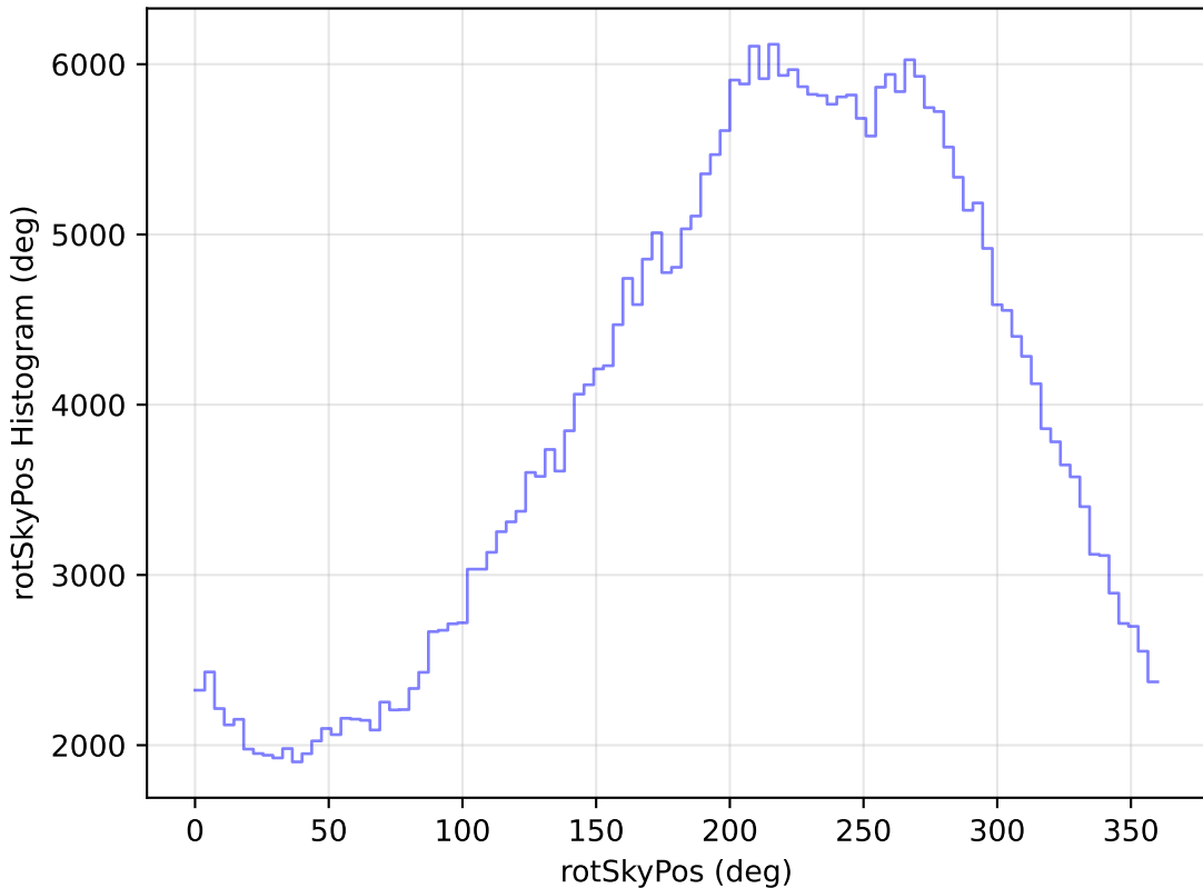
too_elab_r32_d3_ugrizy_v3.4_10yrs All sky y band: rotSkyPos Histogram
