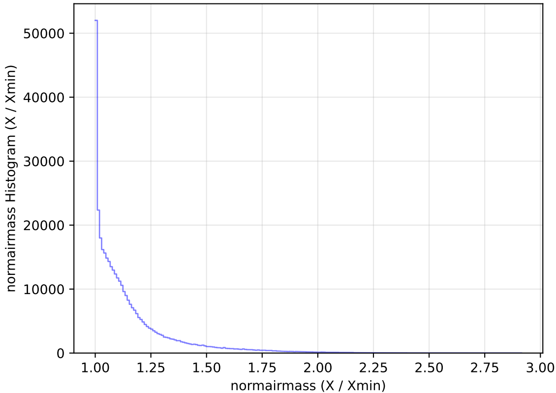
too_elab_r32_d3_ugrizy_v3.4_10yrs WFD y band: normairmass Histogram
