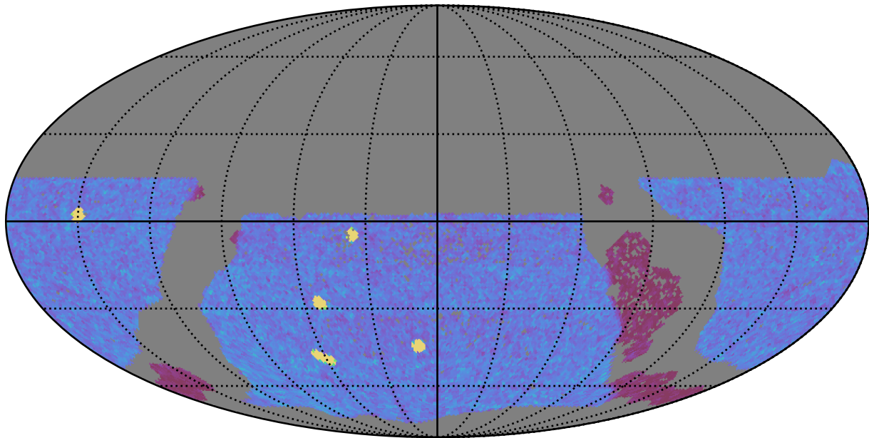
too_elab_r32_d3_ugrizy_v3.4_10yrs WFD y band: NVisits
