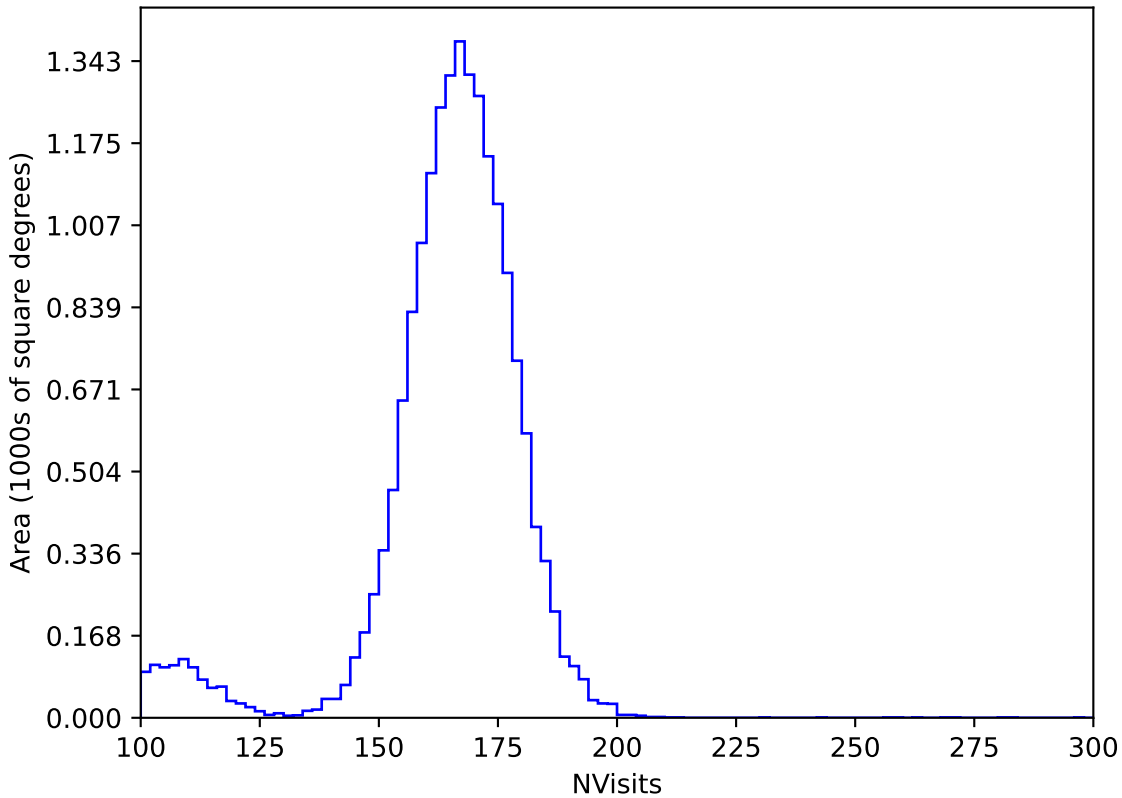
too_elab_r32_d3_ugrizy_v3.4_10yrs WFD y band: NVisits
