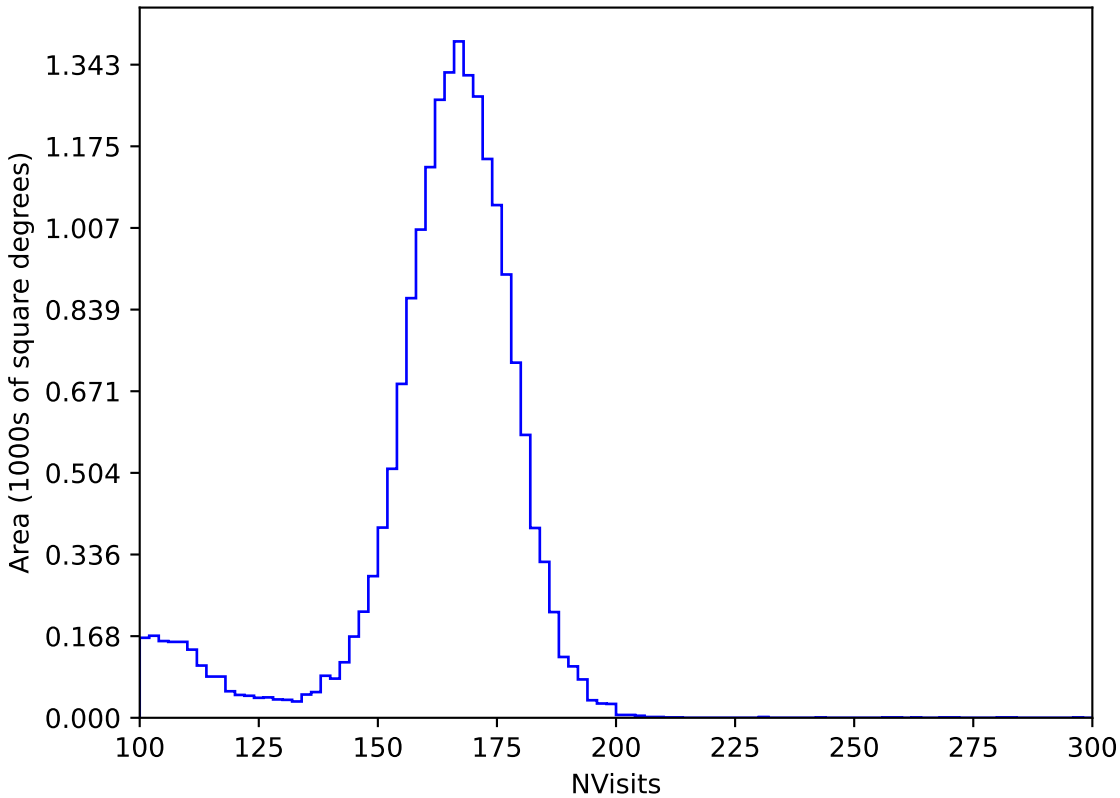
too_elab_r32_d3_ugrizy_v3.4_10yrs All sky y band: NVisits
