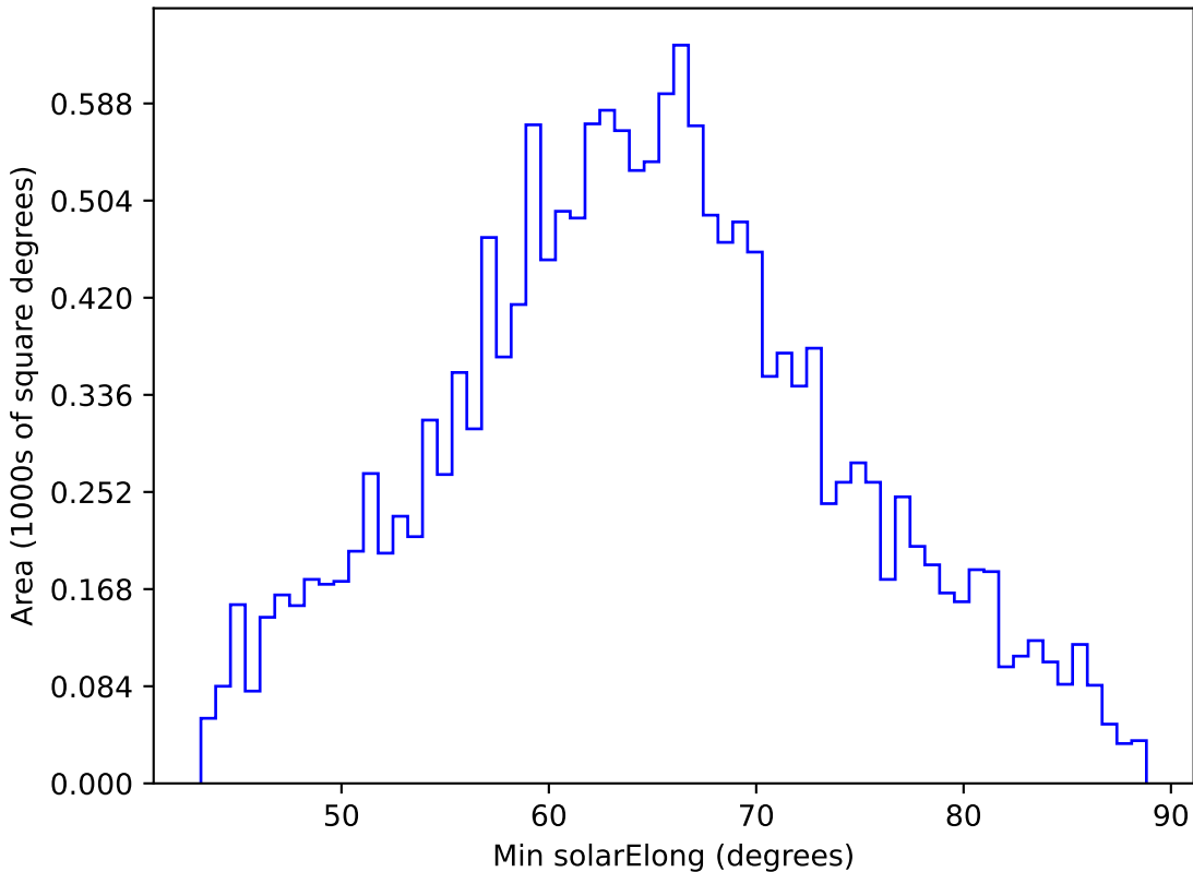
too_elab_r32_d3_ugrizy_v3.4_10yrs WFD y band: Min solarElong
