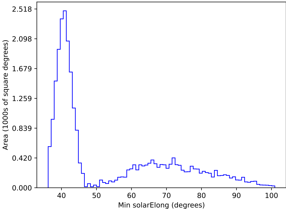
too_elab_r32_d3_ugrizyv3.4_10yrs All sky i band: Min solarElong
