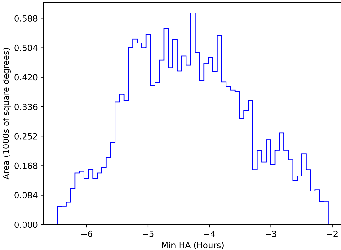
too_elab_r32_d3_ugrizy_v3.4_10yrs WFD z band: Min HA
