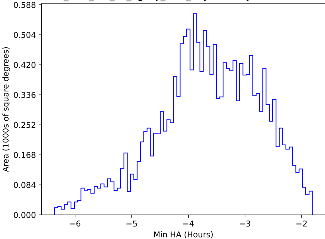
too_elab_r32_d3_ugrizy_v3.4_10yrs WFD y band: Min HA
