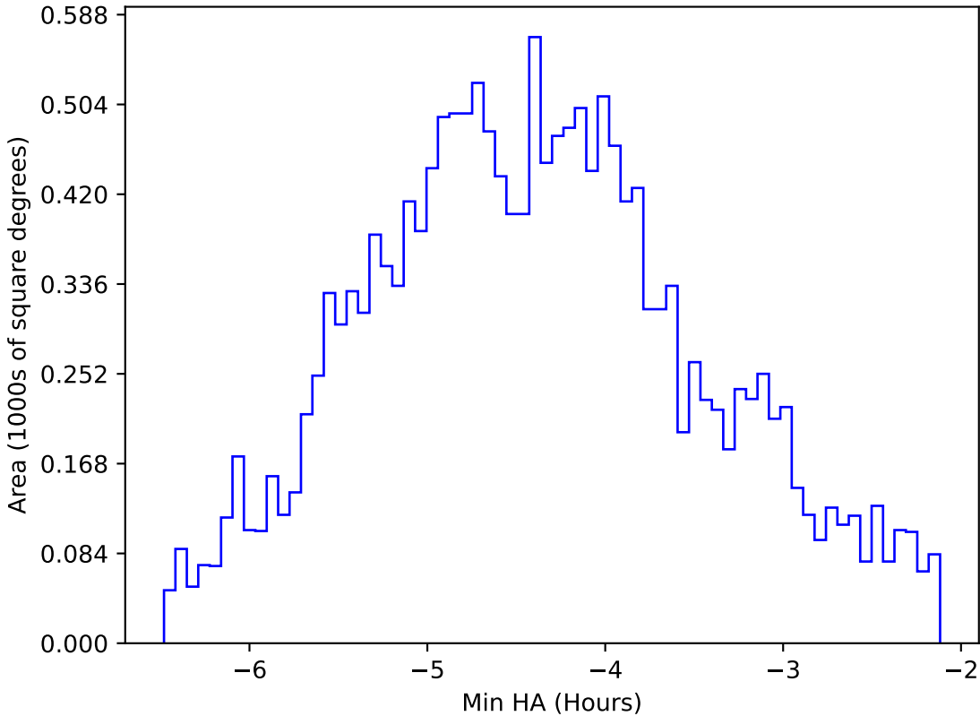
too_elab_r32_d3_ugrizy_v3.4_10yrs WFD i band: Min HA
