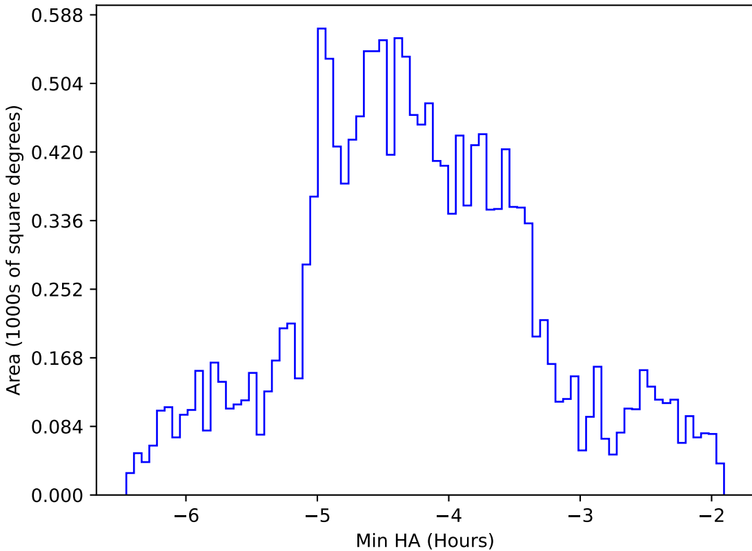
too_elab_r32_d3_ugrizy_v3.4_10yrs WFD g band: Min HA
