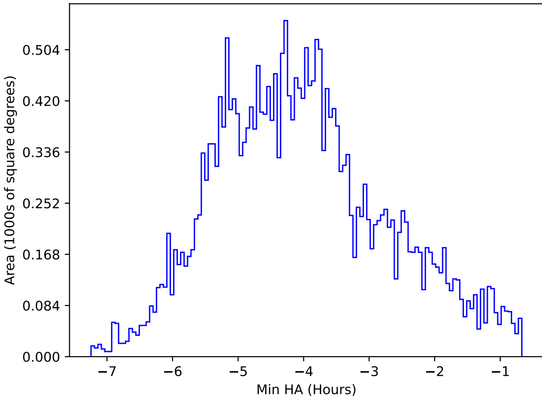
too_elab_r32_d3_ugrizy_v3.4_10yrs All sky z band: Min HA
