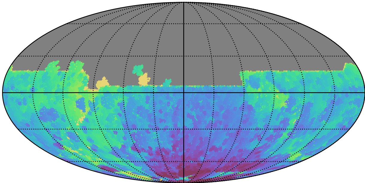
too_elab_r32_d3_ugrizy_v3.4_10yrs All sky y band: Min HA
