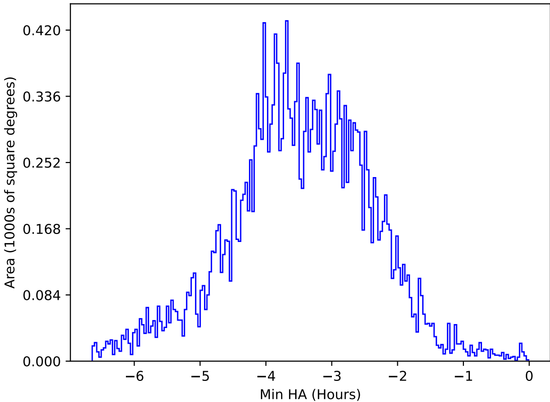
too_elab_r32_d3_ugrizy_v3.4_10yrs All sky y band: Min HA
