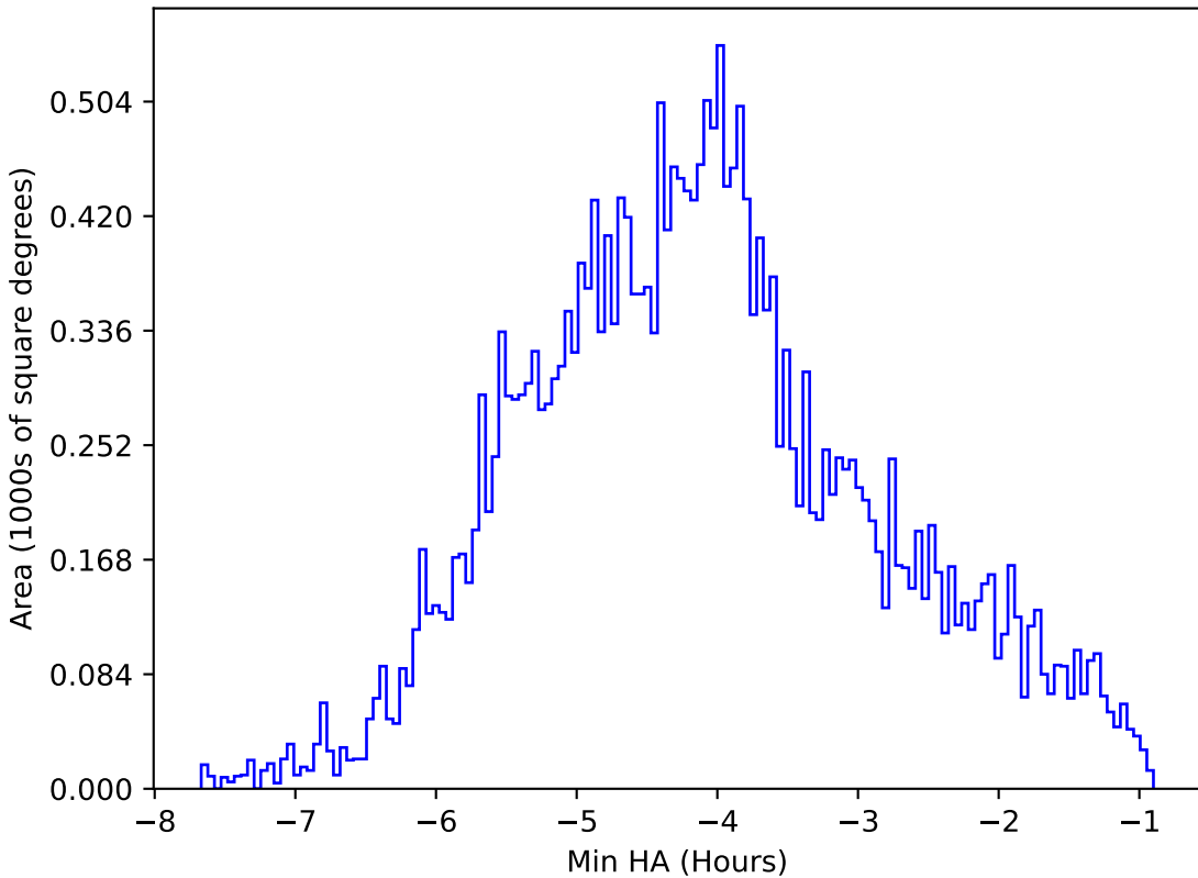
too_elab_r32_d3_ugrizy_v3.4_10yrs All sky i band: Min HA
