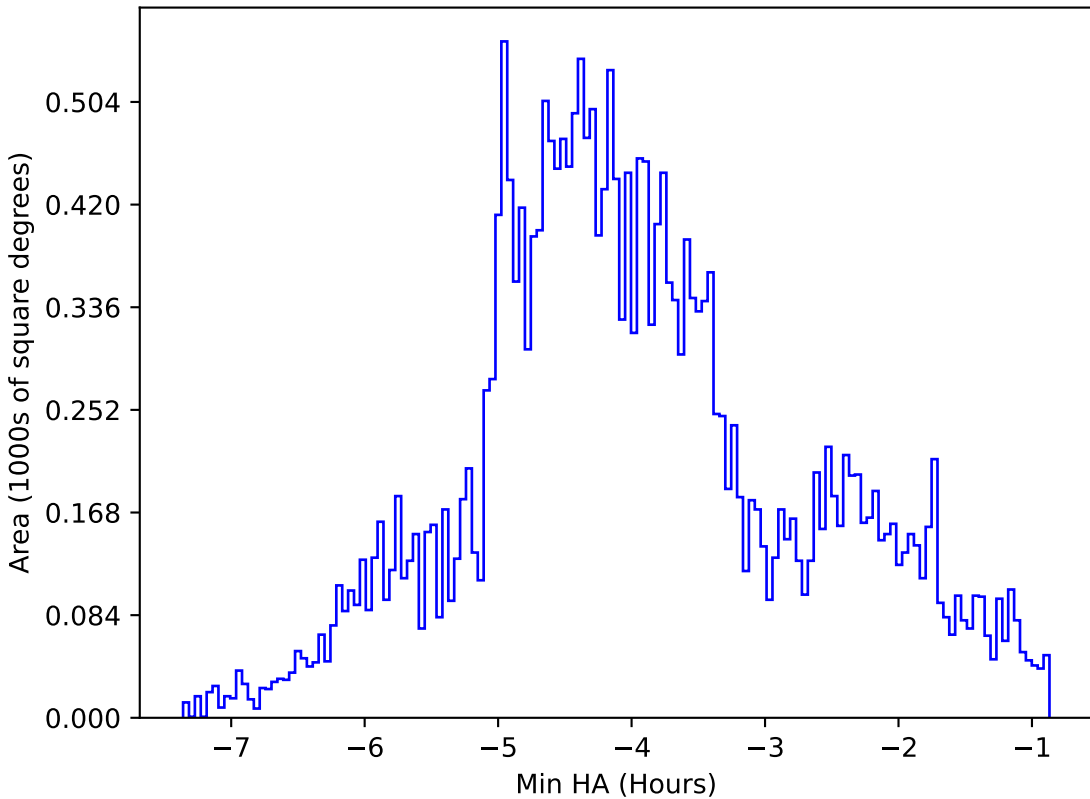
too_elab_r32_d3_ugrizy_v3.4_10yrs All sky g band: Min HA
