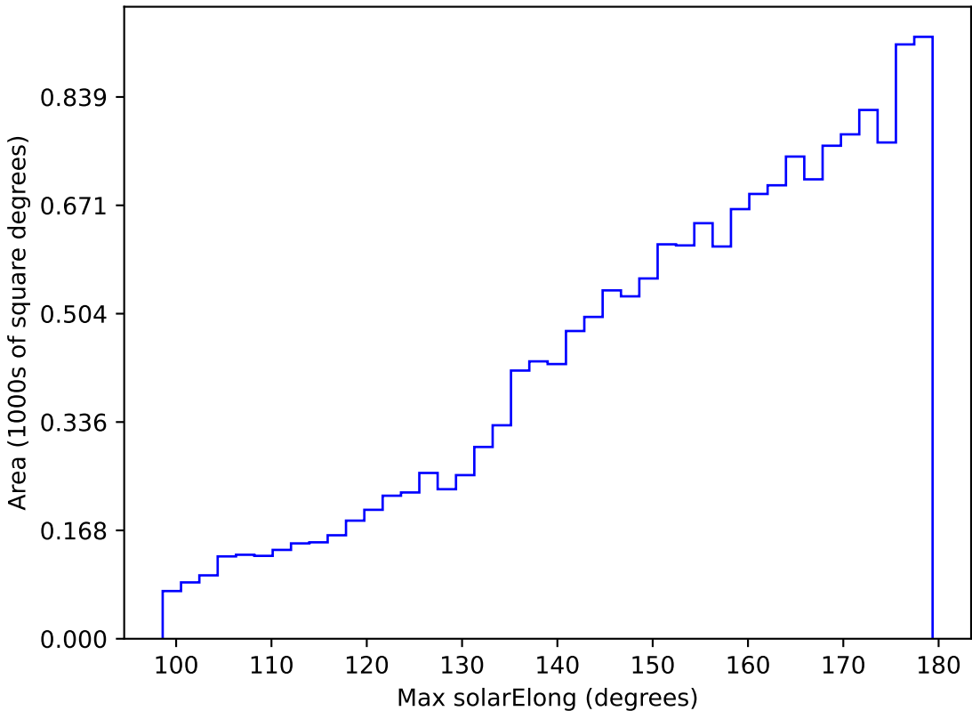
too_elab_r32_d3_ugrizy_v3.4_10yrs WFD y band: Max solarElong
