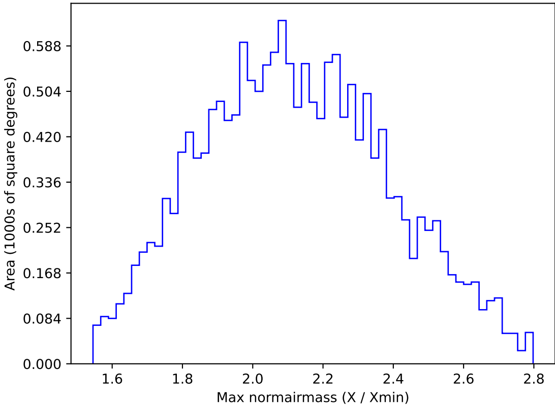
too_elab_r32_d3_ugrizy_v3.4_10yrs WFD y band: Max normairmass
