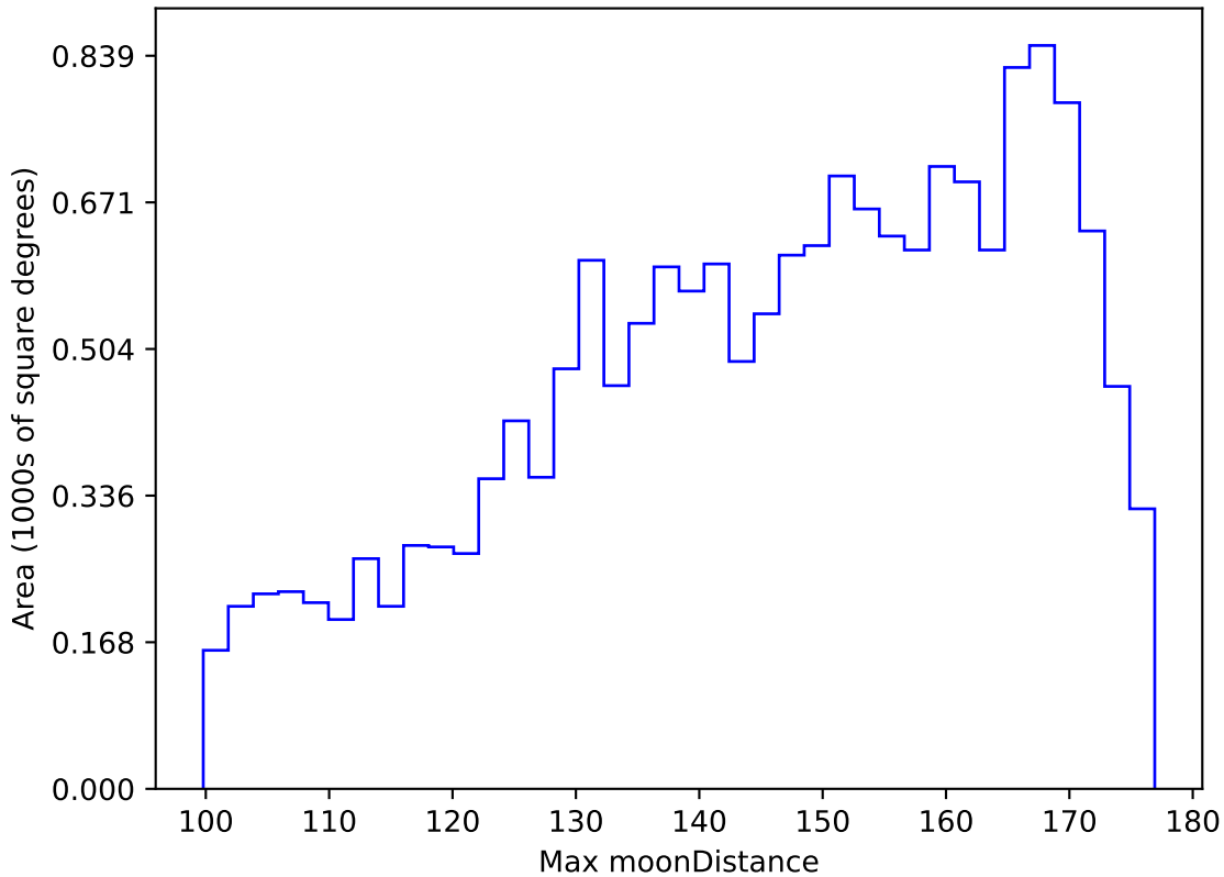
too_elab_r32_d3_ugrizy_v3.4_10yrs WFD y band: Max moonDistance
