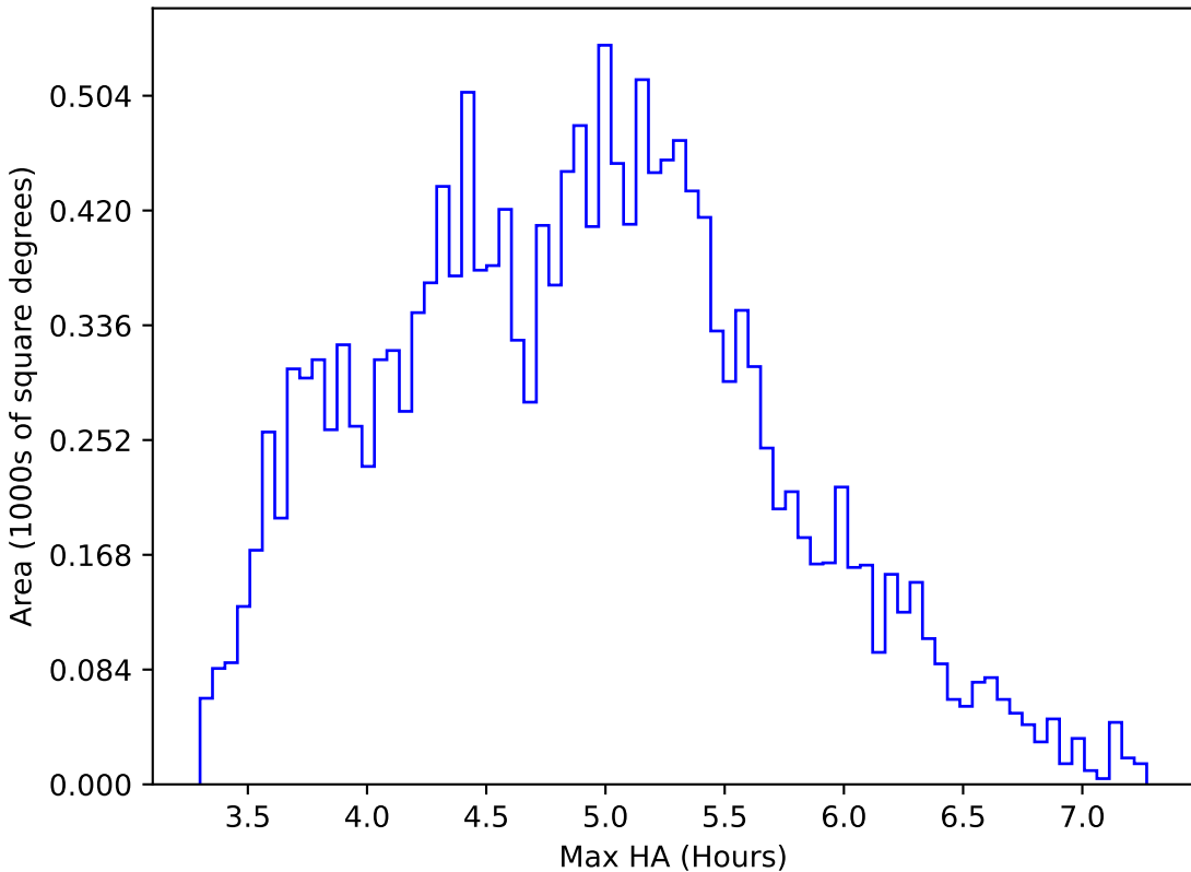
too_elab_r32_d3_ugrizy_v3.4_10yrs WFD z band: Max HA
