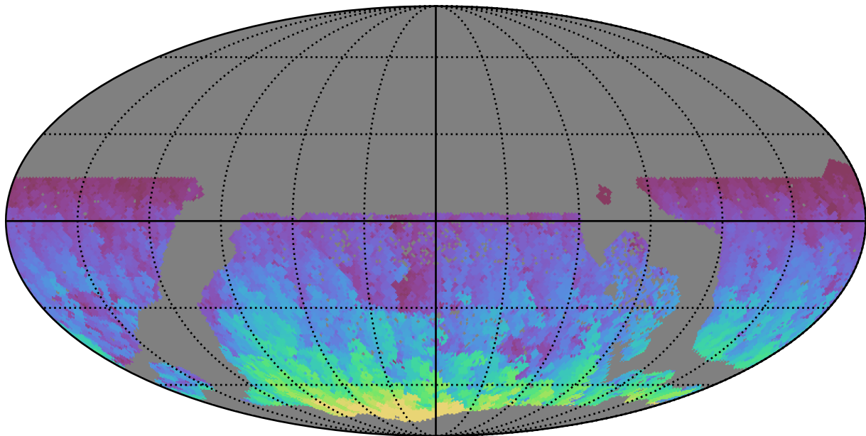
too_elab_r32_d3_ugrizy_v3.4_10yrs WFD y band: Max HA
