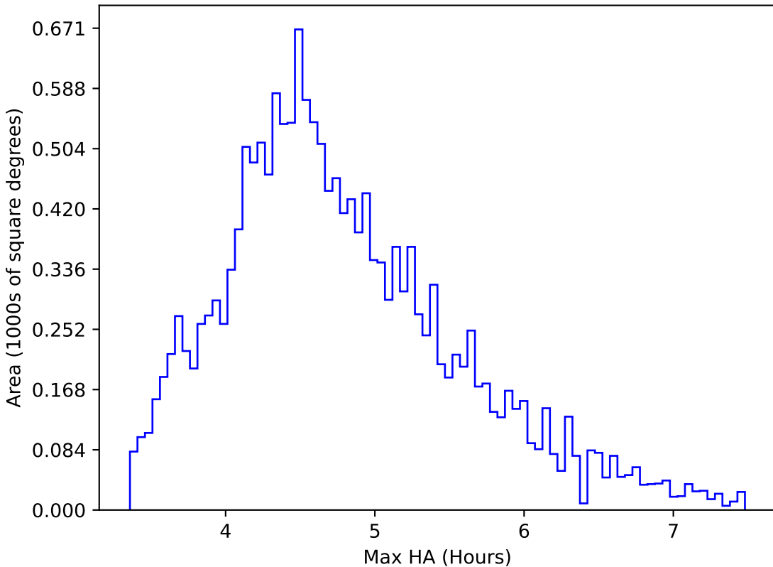
too_elab_r32_d3_ugrizy_v3.4_10yrs WFD y band: Max HA
