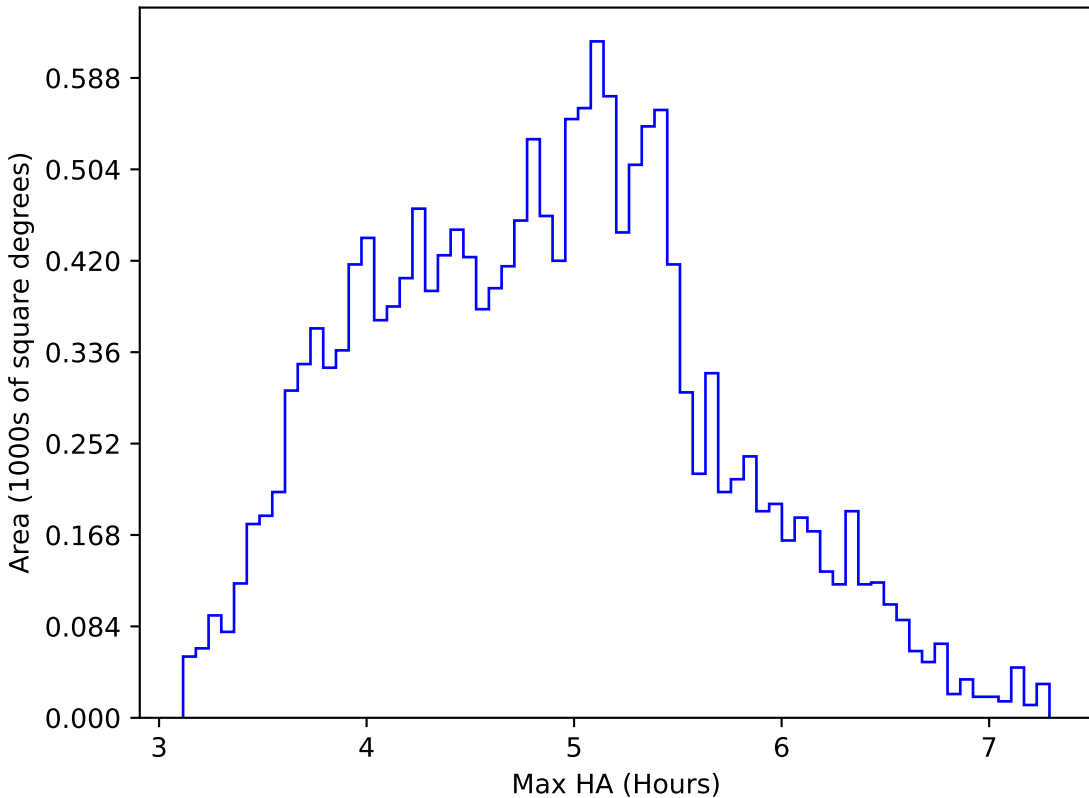
too_elab_r32_d3_ugrizy_v3.4_10yrs WFD i band: Max HA
