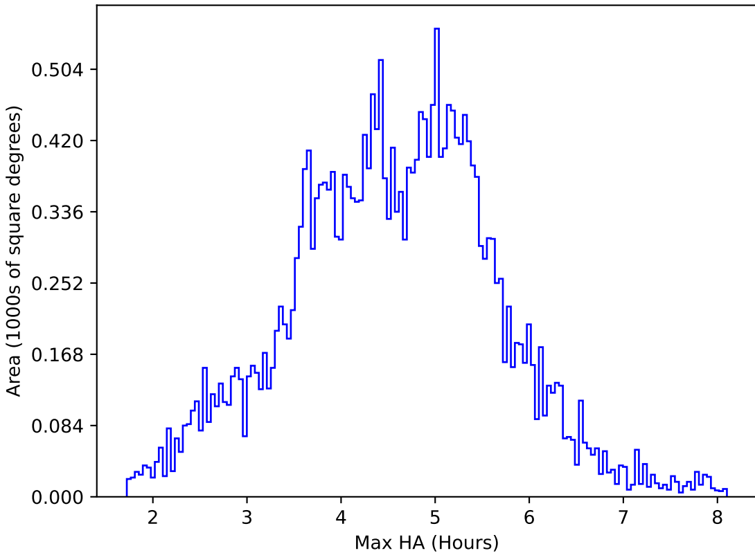
too_elab_r32_d3_ugrizy_v3.4_10yrs All sky z band: Max HA
