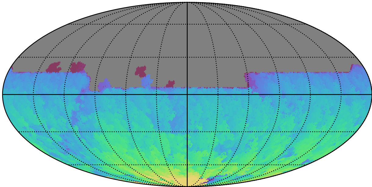
too_elab_r32_d3_ugrizy_v3.4_10yrs All sky y band: Max HA
