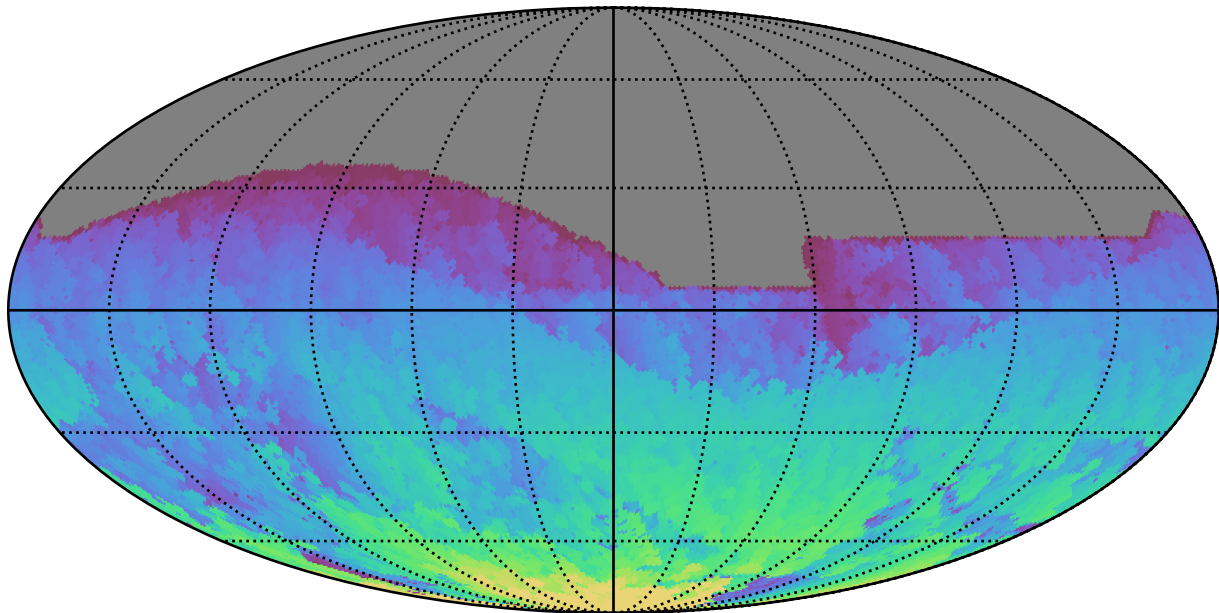
too_elab_r32_d3_ugrizy_v3.4_10yrs All sky i band: Max HA
