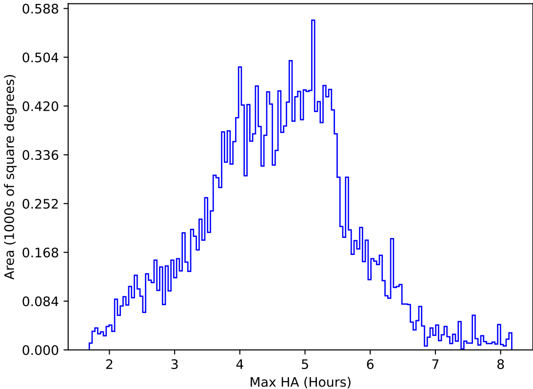
too_elab_r32_d3_ugrizy_v3.4_10yrs All sky i band: Max HA
