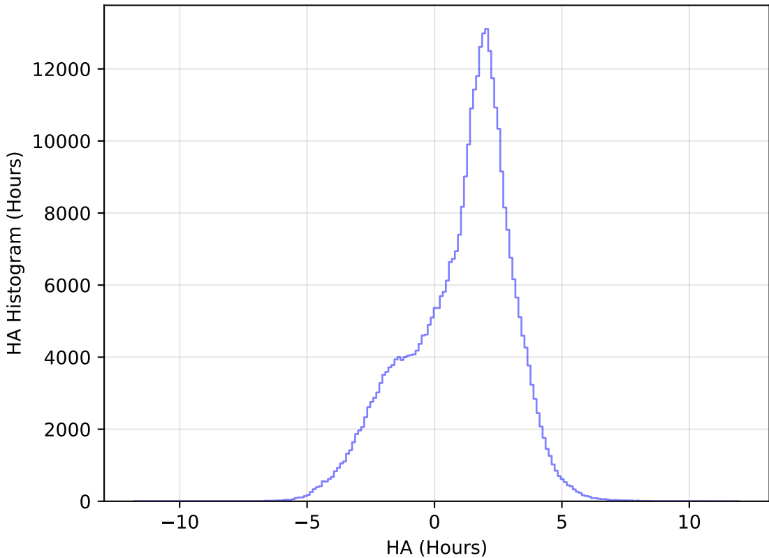
too_elab_r32_d3_ugrizy_v3.4_10yrs All sky y band: HA Histogram
