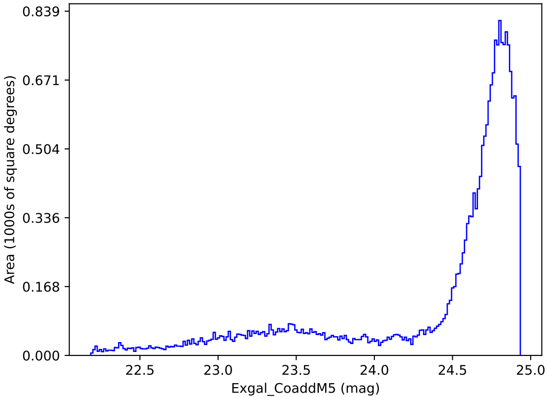
too_elab_r32_d3_ugrizy_v3.4_10yrs All sky y band: Exgal_CoaddM5
