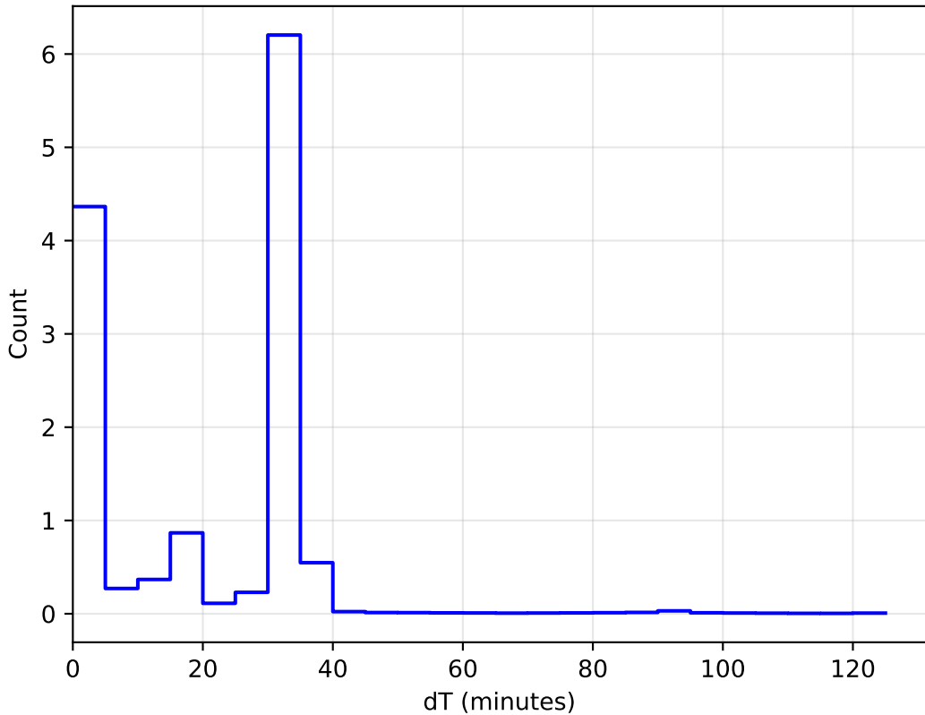
too_elab_r32_d3_ugrizy_v3.4_10yrs All sky: DeltaT Histogram 1e6
