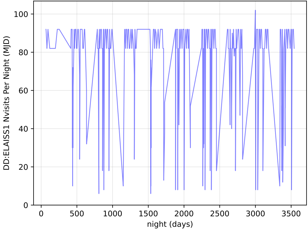
too_elab_r32_d3_ugrizy_v3.4_10yrs all bands: DD:ELAISS1 Nvisits Per Night
