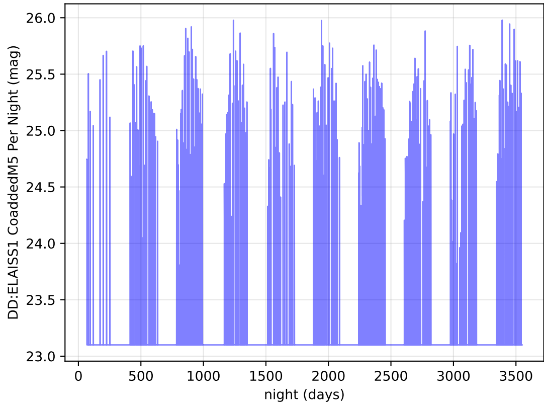
too_elab_r32_d3_ugrizy_v3.4_10yrs i band: DD:ELAISS1 CoaddedM5 Per Night
