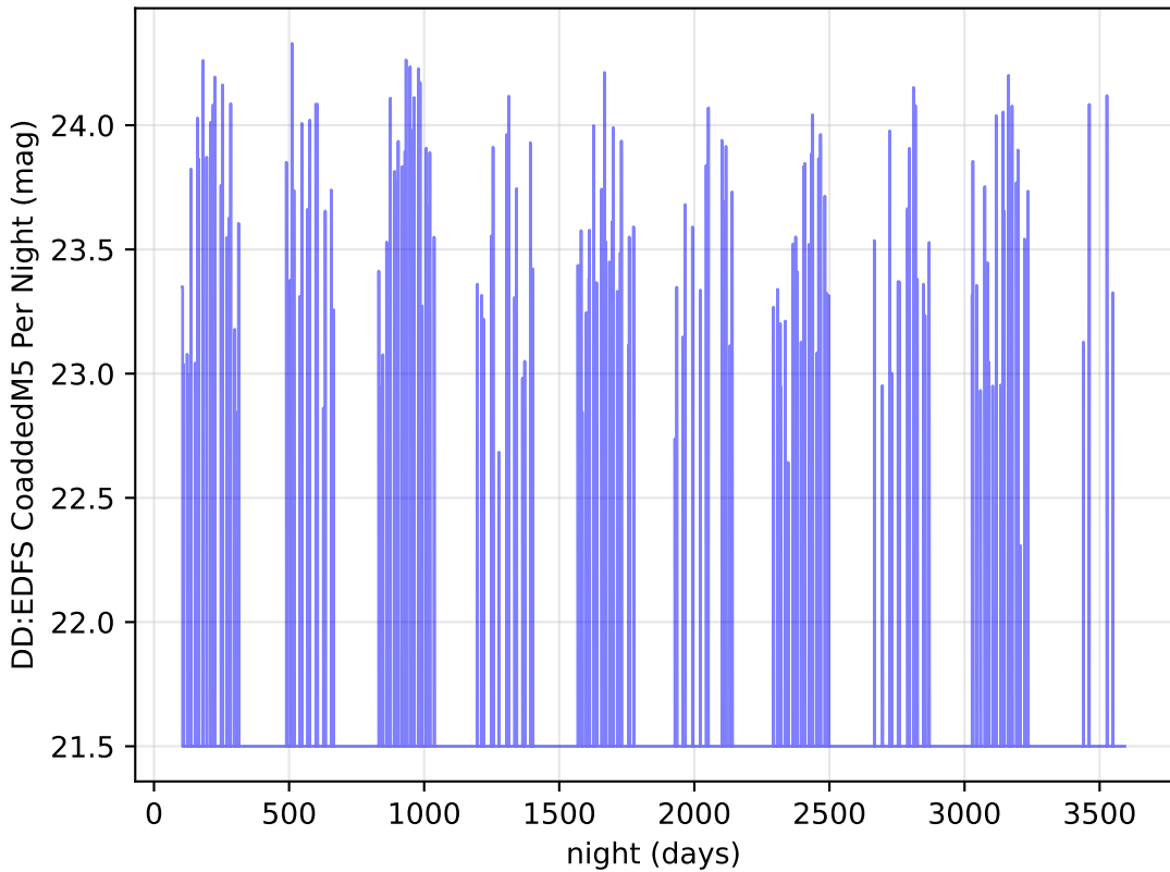
too_elab_r32_d3_ugrizy_v3.4_10yrs y band: DD:EDFS CoaddedM5 Per Night
