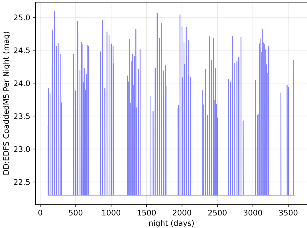
too_elab_r32_d3_ugrizy_v3.4_10yrs u band: DD:EDFS CoaddedM5 Per Night
