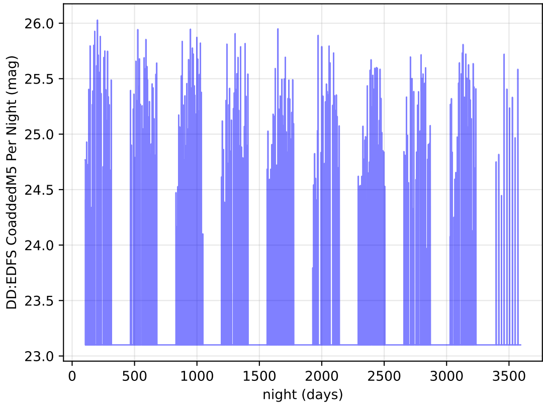
too_elab_r32_d3_ugrizy_v3.4_10yrs i band: DD:EDFS CoaddedM5 Per Night
