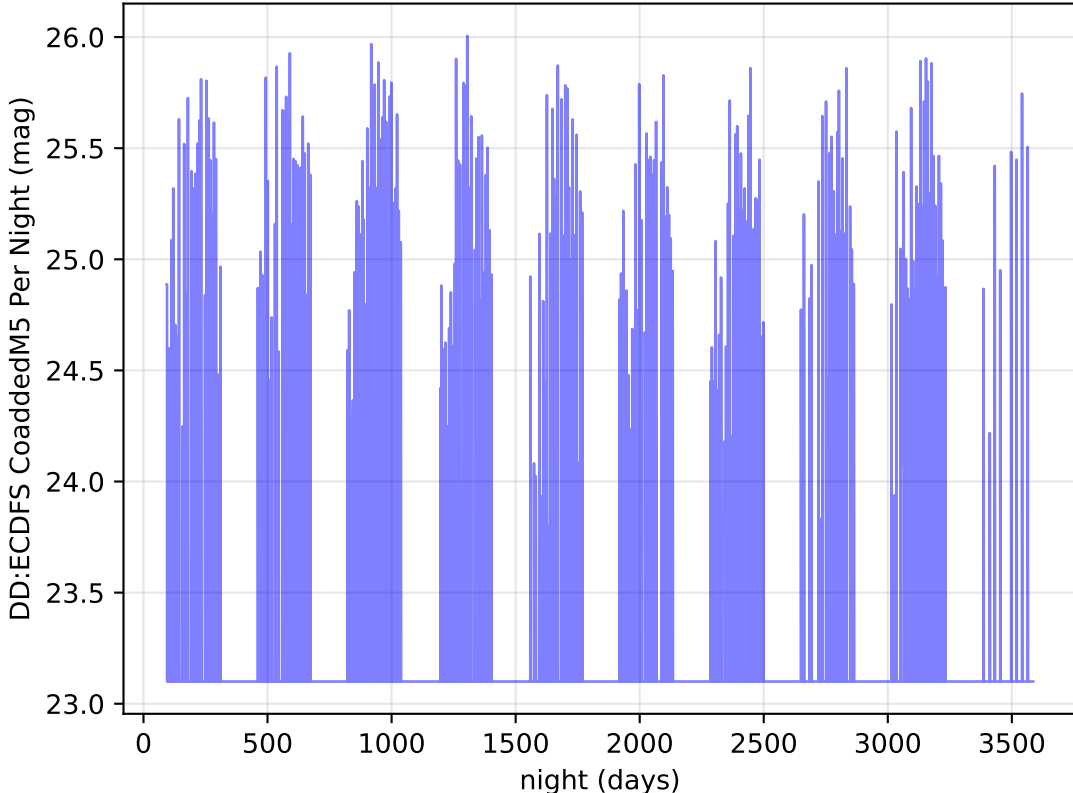
too_elab_r32_d3_ugrizy_v3.4_10yrs i band: DD:ECDFS CoaddedM5 Per Night
