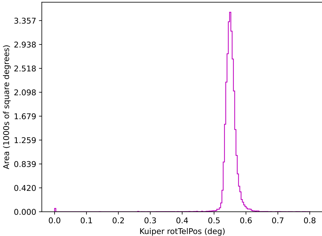
too_elab_r32_d3_gz_v3.4_10yrs z: Kuiper rotTelPos
