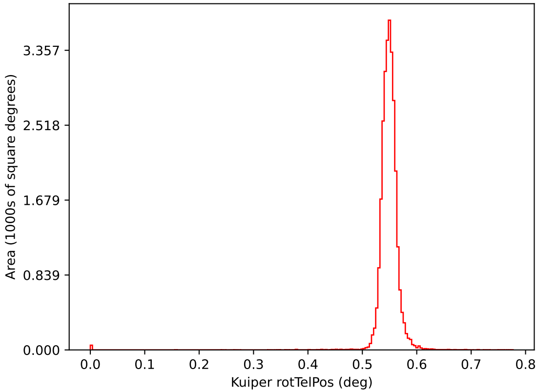
too_elab_r32_d3_gz_v3.4_10yrs i: Kuiper rotTelPos
