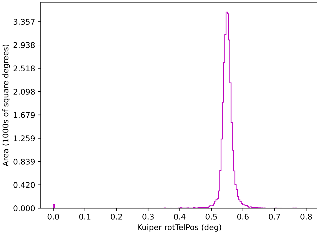
too_elab_r32_d3_griz_v3.4_10yrs z: Kuiper rotTelPos
