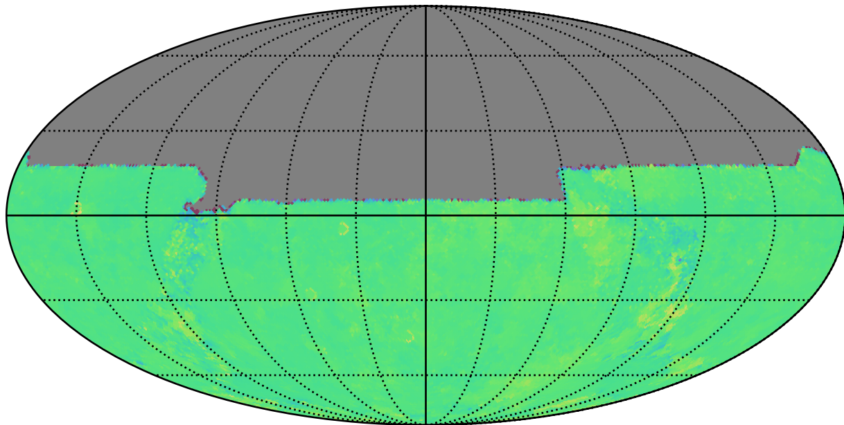
too_elab_r32_d3_griz_v3.4_10yrs u: Kuiper rotTelPos
