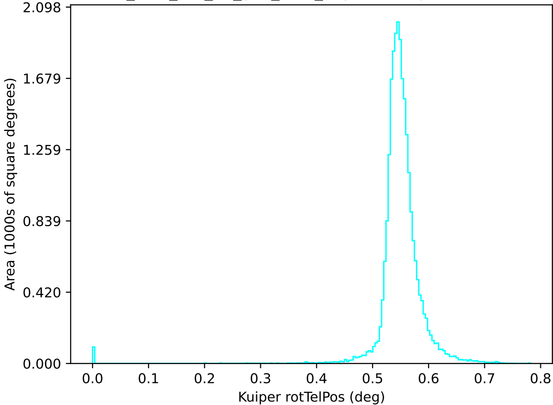
too_elab_r32_d3_griz_v3.4_10yrs u: Kuiper rotTelPos
