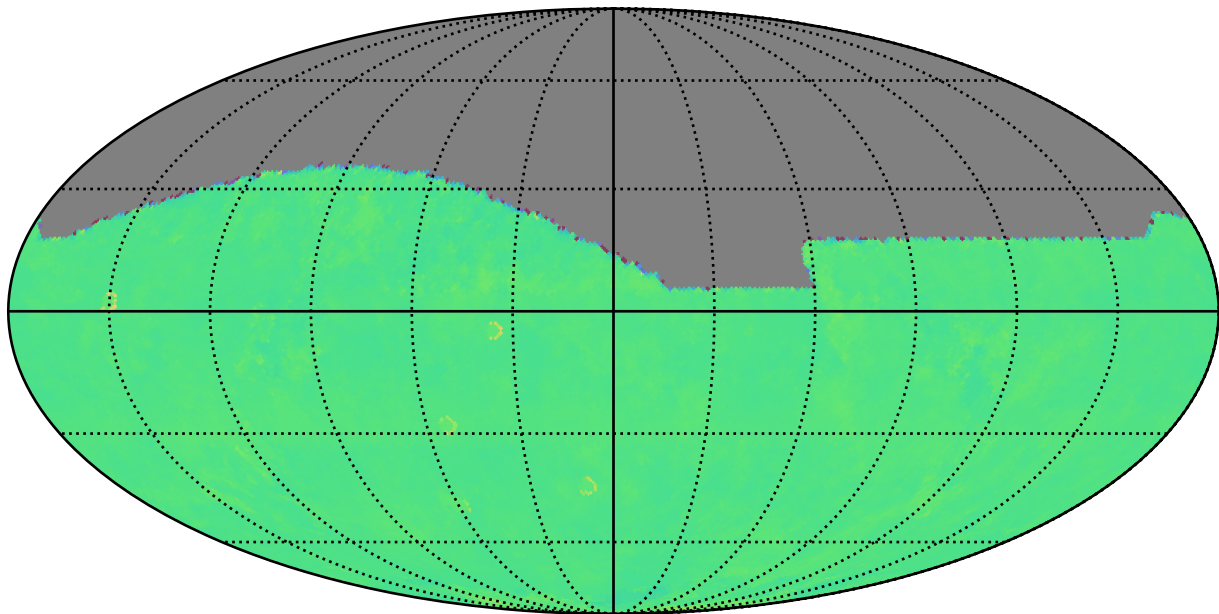
too_elab_r32_d3_griz_v3.4_10yrs i: Kuiper rotTelPos
