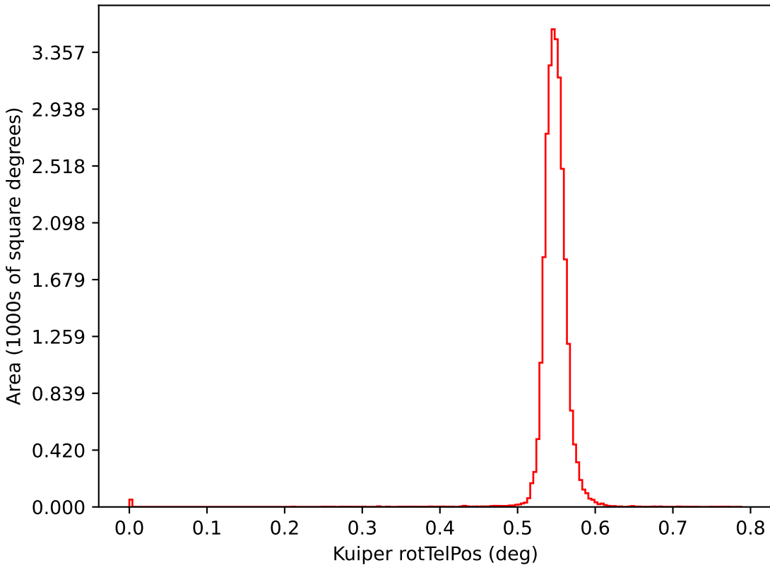
too_elab_r32_d3_griz_v3.4_10yrs i: Kuiper rotTelPos
