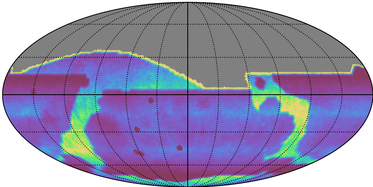
too_elab_r32_d3_griz_v3.4_10yrs : DCRprecision
