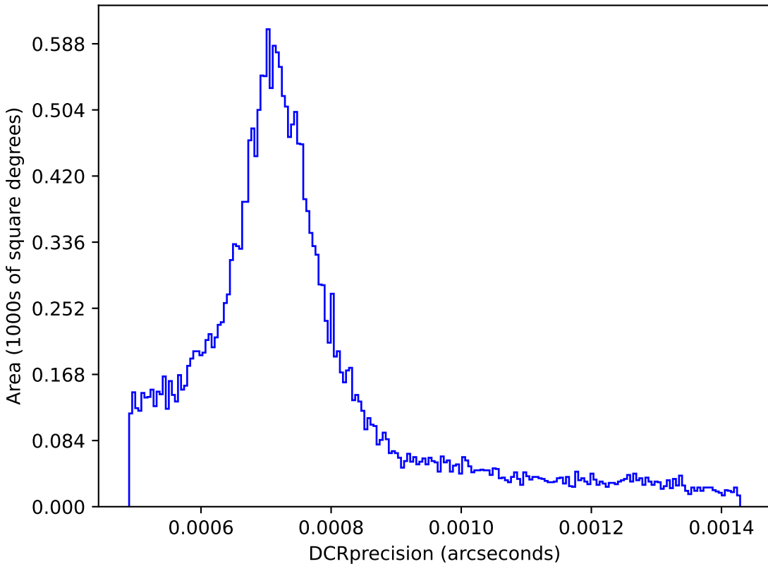
too_elab_r32_d3_griz_v3.4_10yrs : DCRprecision
