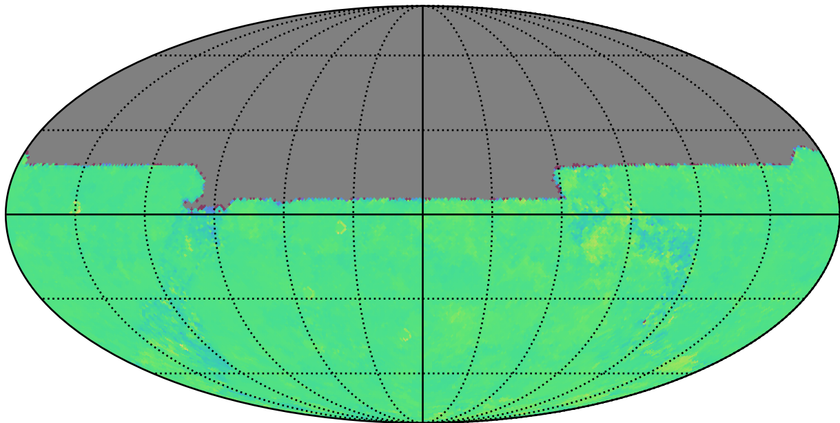
too_elab_r32_d3_giz_v3.4_10yrs u: Kuiper rotTelPos
