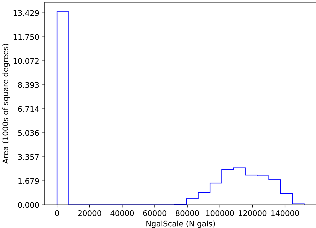
too_elab_r32_d2_ugrizy_v3.4_10yrs i: NgalScale
