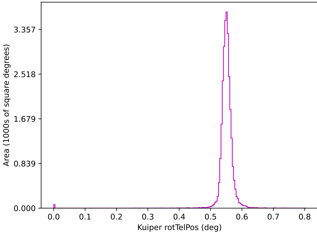
too_elab_r32_d2_ugrizy_v3.4_10yrs z: Kuiper rotTelPos
