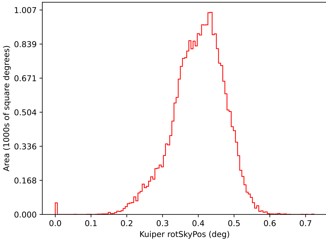
too_elab_r32_d2_ugrizy_v3.4_10yrs i: Kuiper rotSkyPos
