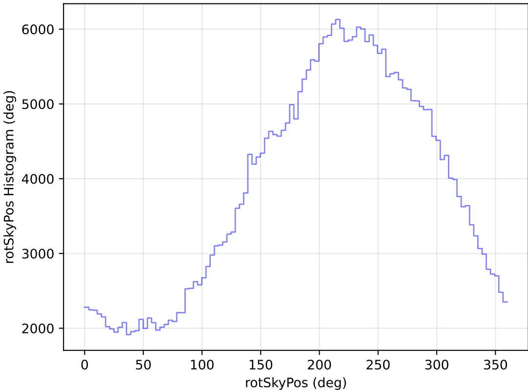
too_elab_r32_d2_ugrizy_v3.4_10yrs WFD y band: rotSkyPos Histogram
